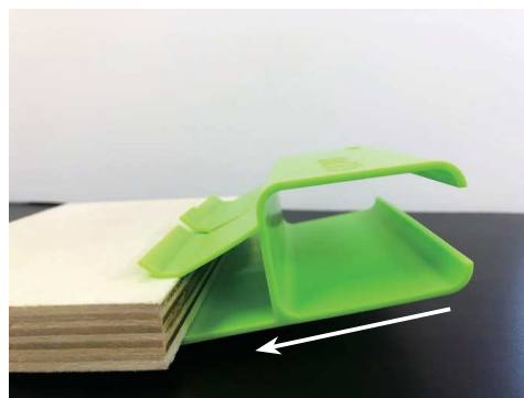
② カチットⅡを少し斜めに傾け、抜型へ少し差し込みます
